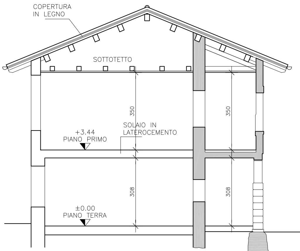
SEZIONE A-A
