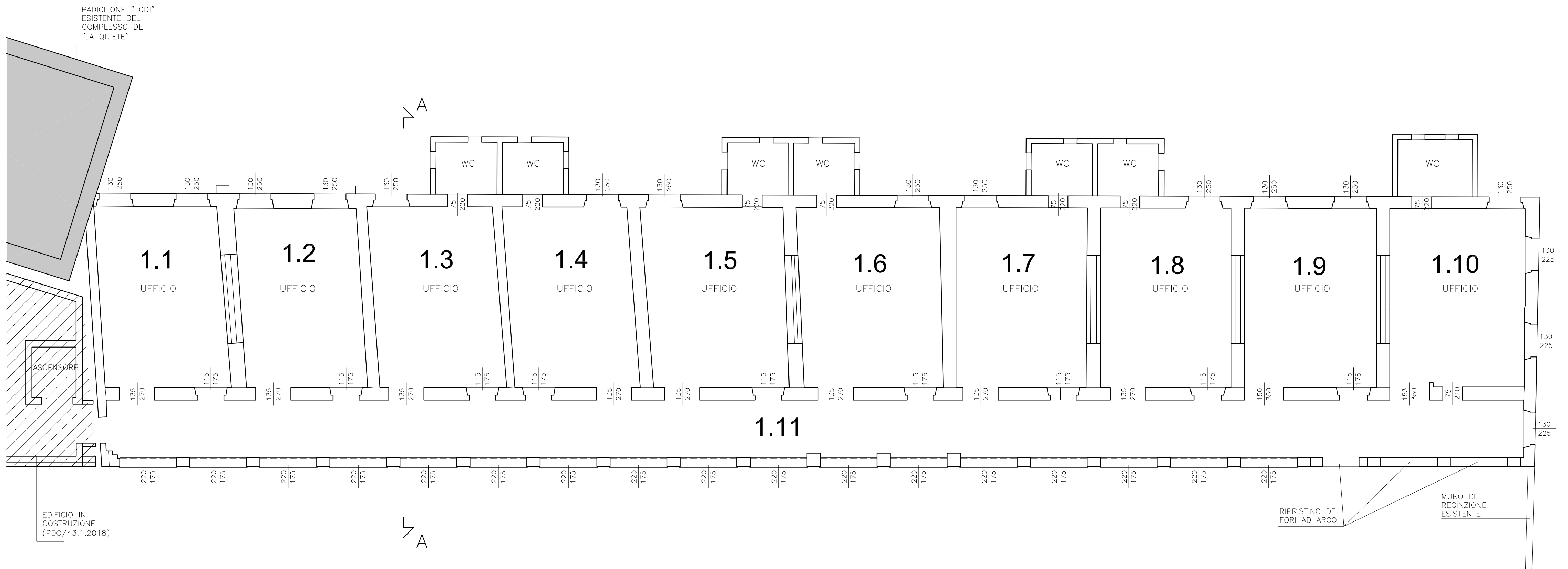
PIANO PRIMO 1:100
