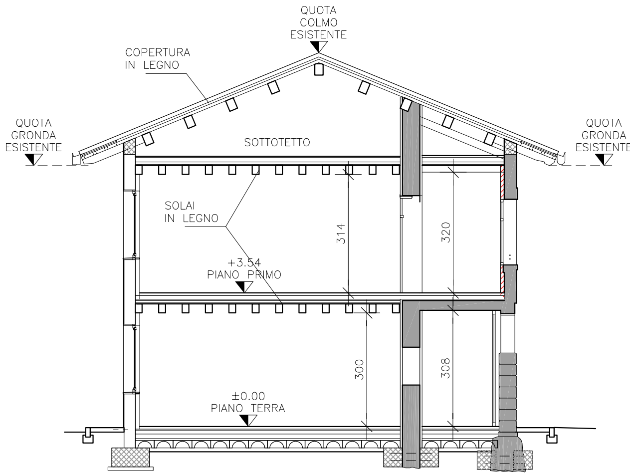
SEZIONE A-A
