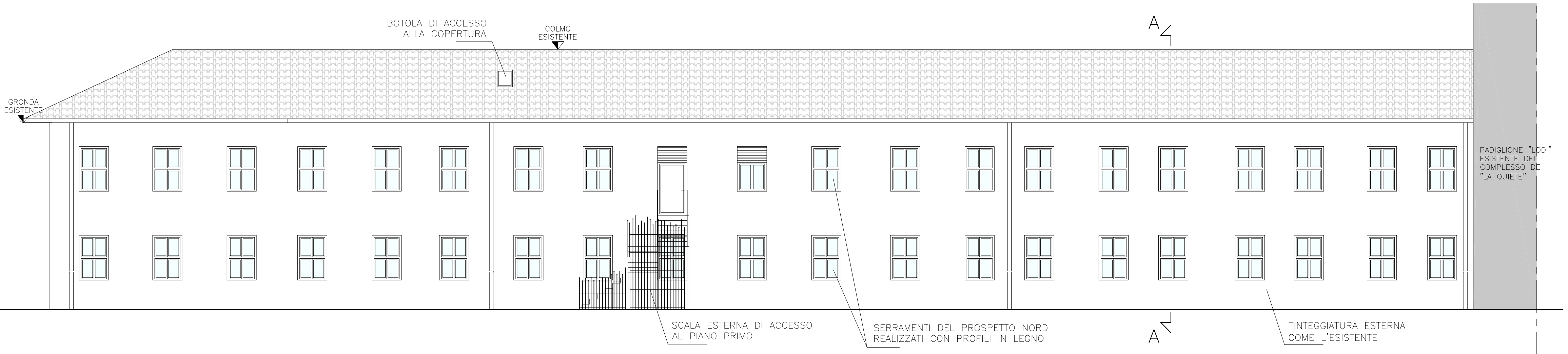
PROSPETTO NORD
