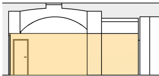
Sezione A-A'
