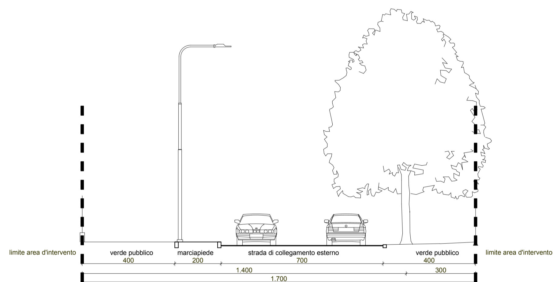
SEZIONE A-A
