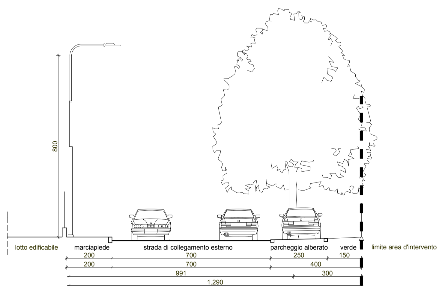
SEZIONE B-B
