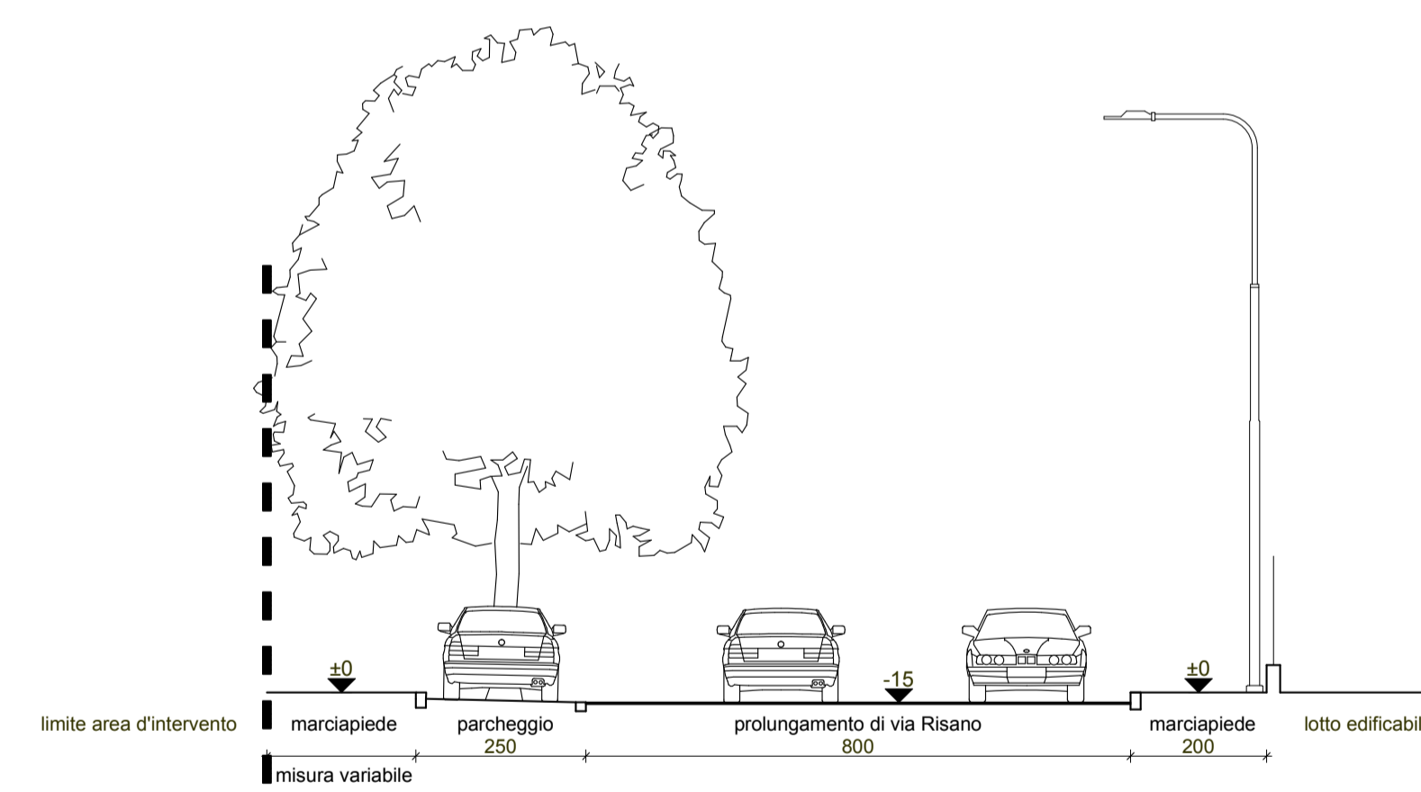
SEZIONE D-D
